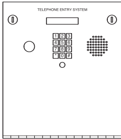
1803 Surface 11.25" W x 13" H x 4.75" D 28.5cm W x 33cm H x 12cm D
